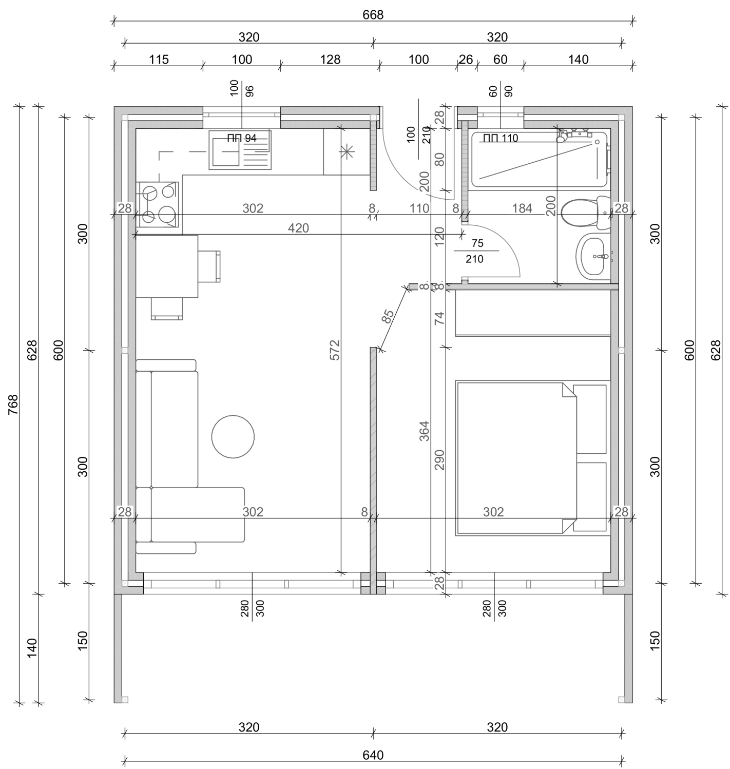
План 1:50
