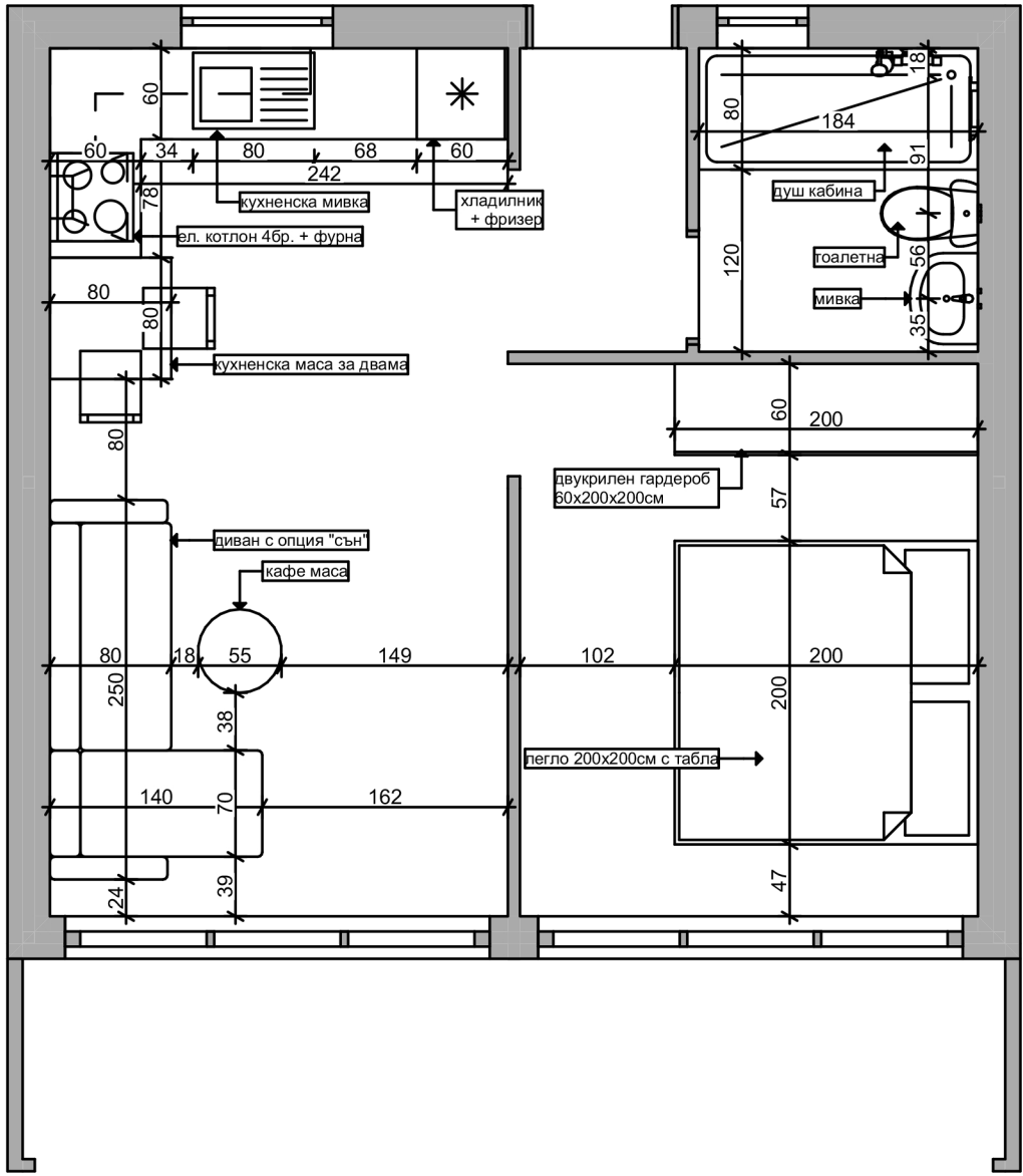
Обзавеждане 1:50
