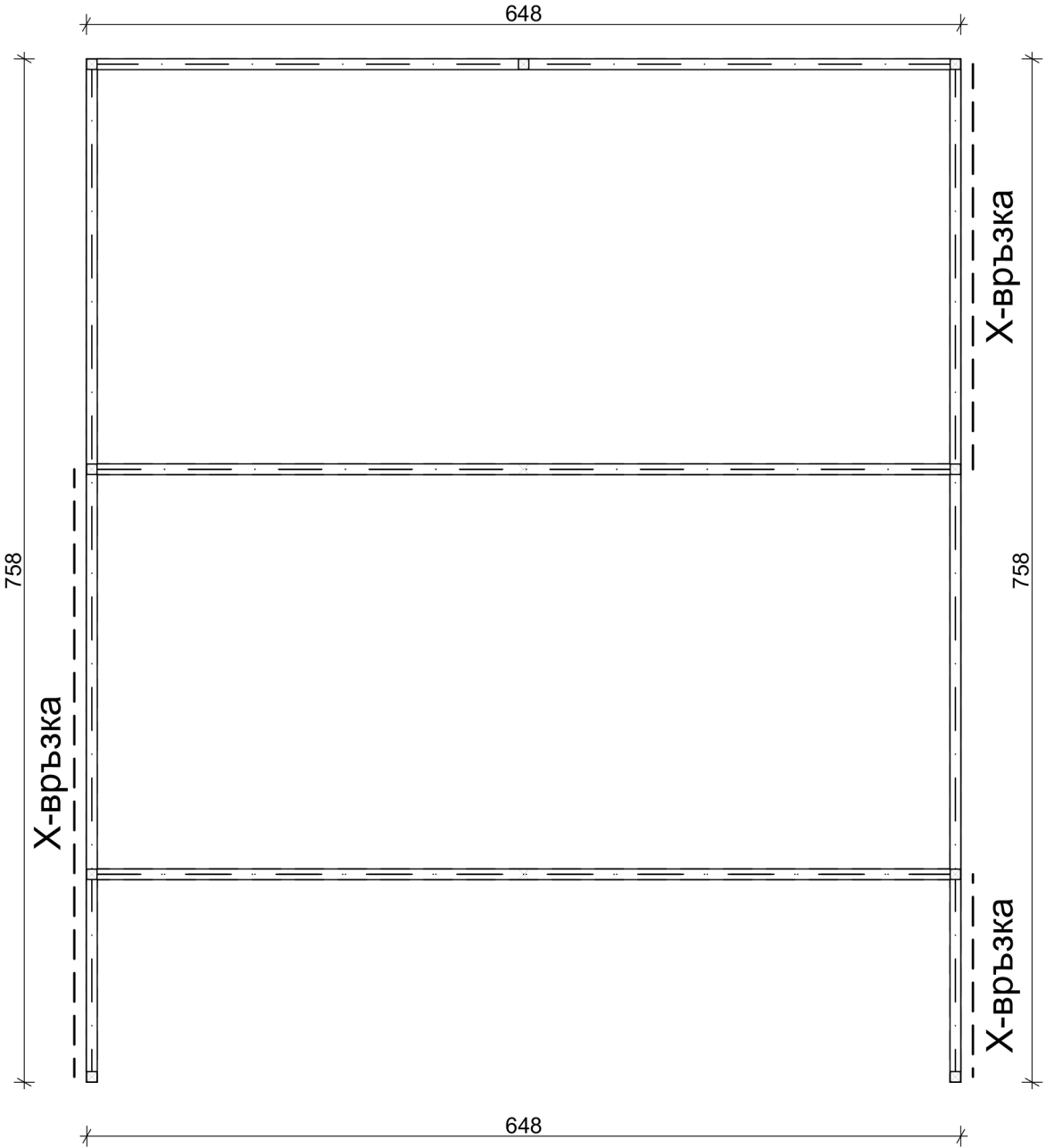
План метална носеща конструкция +0,00 / +3,00 1:50
