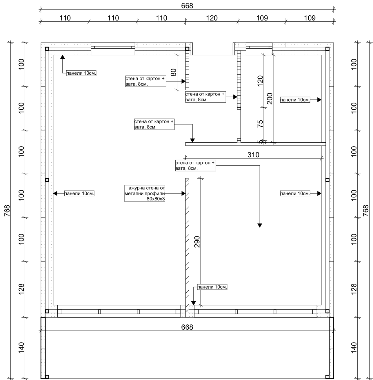
План панели 1:50
