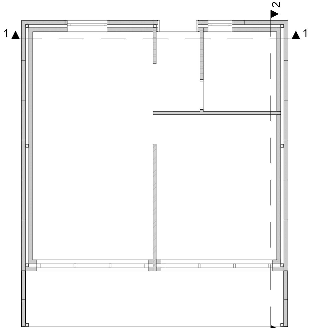
Разрезни линии 1:50
